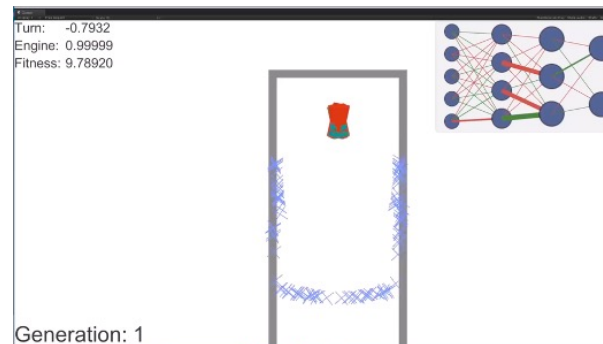
apprentissage automatique
