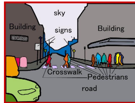
reconnaissance d'objets
